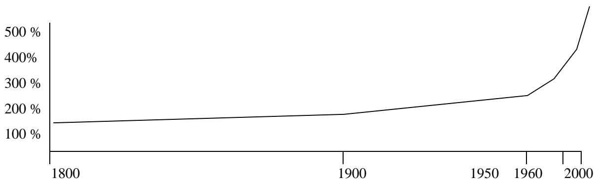
Abb. 5 - 21: Die "Wissensexpllosion"
